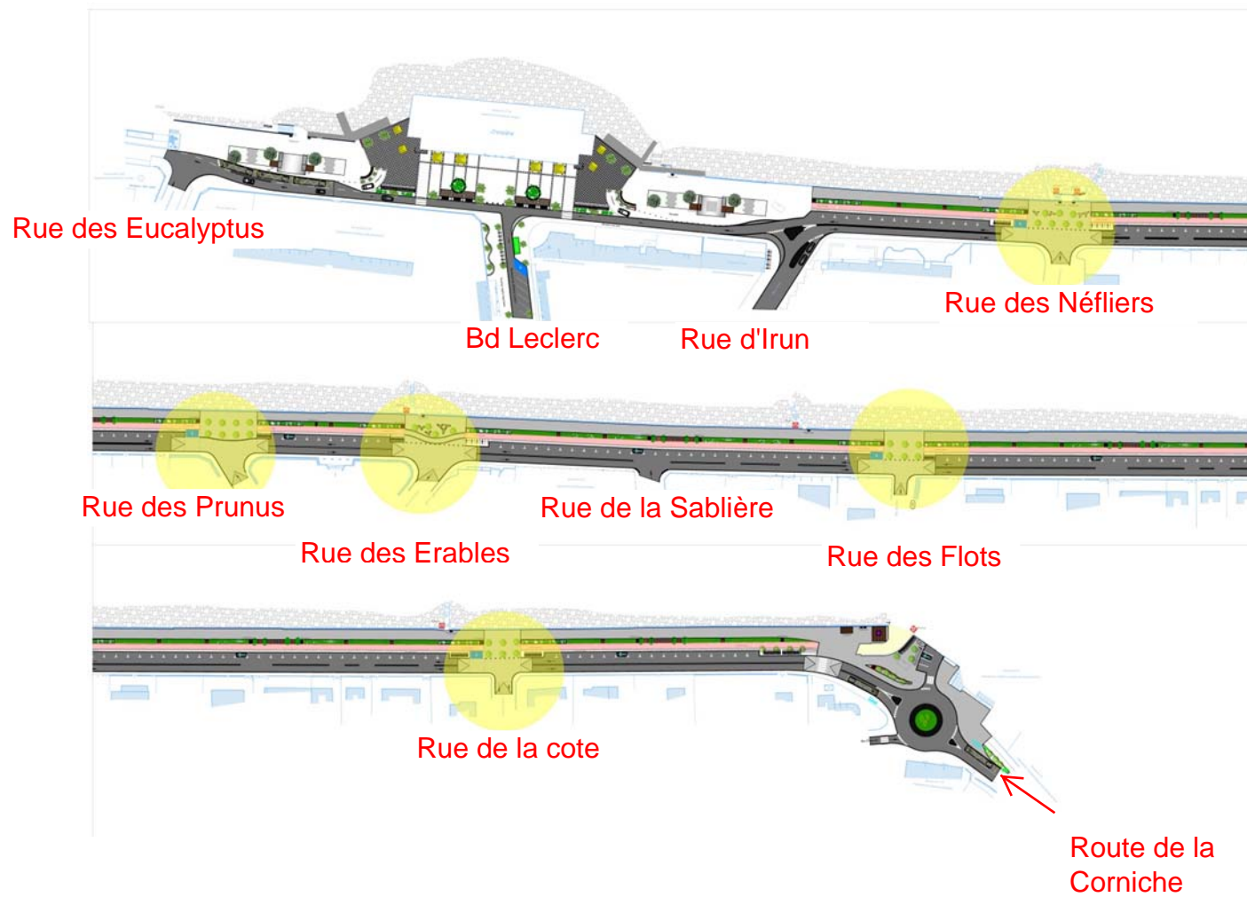
Présentation de principe de voirie en arrivant de la route de la Corniche jusqu'à la station multimodale.
